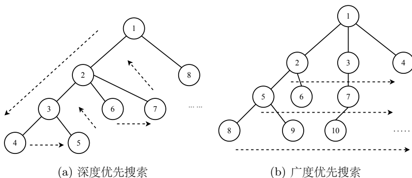
图 15.17: 深度和广度优先搜索的顺序
