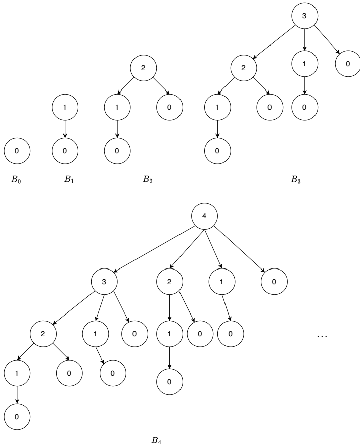
图 10.2: 秩为 0、1、2、3、4……的二项式树
