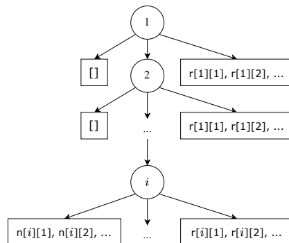
图 12.9: 不规则树, 第 i 层子树的 f 不空
