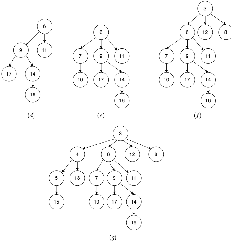
图 10.11: 从右向左合并的步骤:(d) 合并子树 9 和 6;(e) 合并子树 7;(f) 合并子树 3;(g) 合并子树 4。
