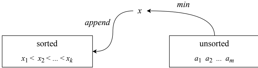
图 9.1: 左侧部分为已序元素,不断从剩余部分选择最小元素附加在左侧尾部
