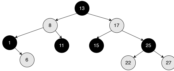
图 4.5: 隐藏 NIL 节点
