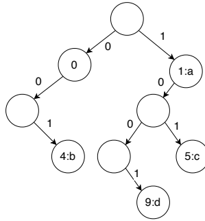
图 6.3: 小端整数 trie, 包含映射: \{1 \rightarrow a, 4 \rightarrow b, 5 \rightarrow c, 9 \rightarrow d\}
