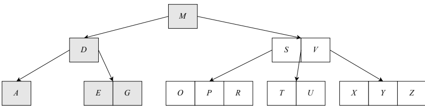
图 7.12: 删除 'K', 然后删除 'N'
