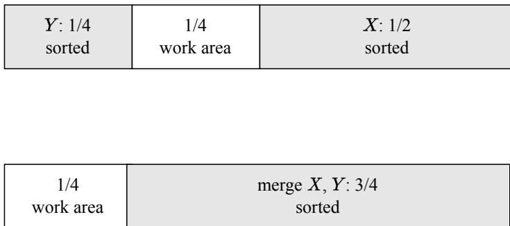
图 13.13: 利用工作区归并 X, Y
