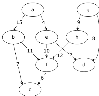
图 15.18: 带权重的有向图
