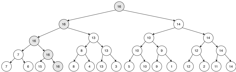
图 9.5: 元素 15 在第一轮就被淘汰
