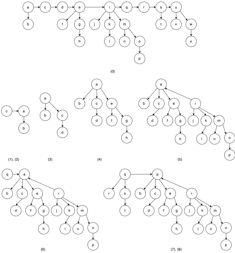
图 10.7: 树归并的步骤。第 3 步, d 先链接到 c, 然后链接到 a; 第 7、8 步, r 先链接到 q, 然后 s 链接到 q。
