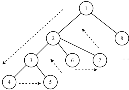
图 15.7: 深度优先搜索的顺序
