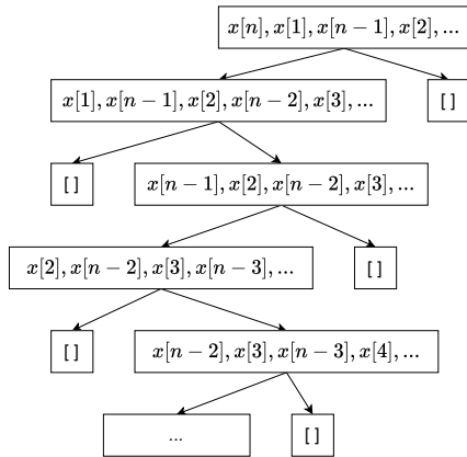
(b) 一个之字形的划分树。
