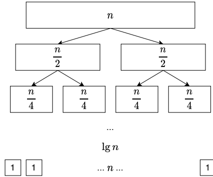
图 13.2: 最好情况, 每次均分。
