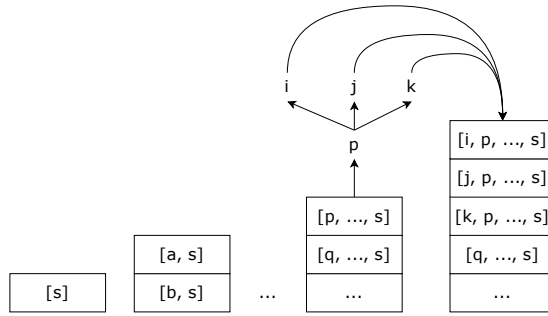
图 15.2: 用栈记录路径
