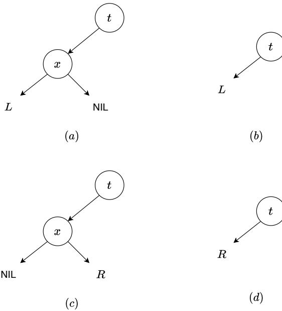
图 2.5: 删除只有一个非空分支的节点
