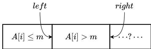
图 1: 数组划分。位于 0 \leq i < left 的元素满足 A[i] \leq m , 位于 left \leq i < right 的元素满足 A[i] > m , 剩余的元素尚未处理。
