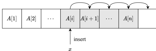
图 3.3: 将元素 x 插入数组 A 中的第 i 个位置
