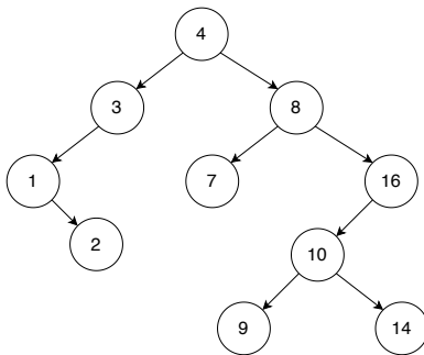
图 2.3: 8 的后继为其右侧分支的最小值 9;为了获得 2 的后继,首先向上找到 1,它没有左子树,继续向上找到 3,3 的左子树也是 2 的祖先,故而后继为 3。
