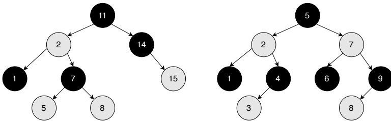
图 4.11: 命令式算法构建出的红黑树
