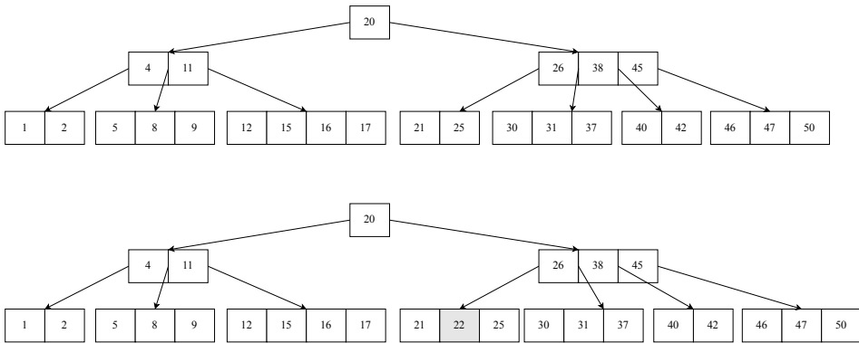
图 7.3: 将 22 插入到 2-3-4 树: 22 > 20 , 插入右子树; 22 < 26 , 插入第一棵子树。 21 < 22 < 25 , 插入到未了的叶子节点。
