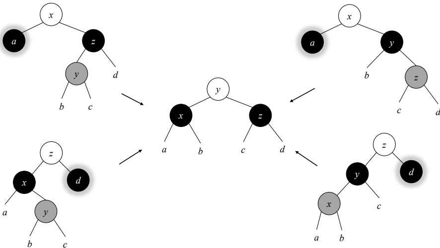
图 A.1: 双重黑色节点的兄弟为黑色,并且该兄弟节点有一个红色子节点。通过一次旋转操作修复。
