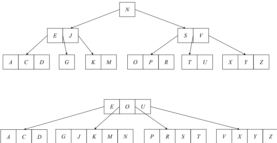
图 7.6: 依次插入“GMPXACDEJKNORSTUVYZ”。
