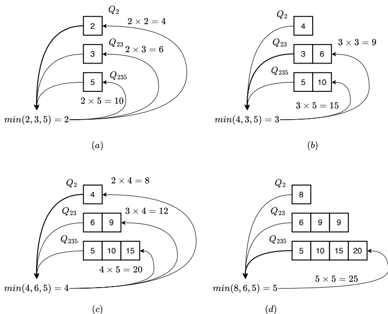
图 4: 使用三个队列 Q_2 、 Q_{23} 、 Q_{235} 构造正规数的前 4 步。
