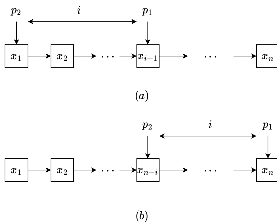
图 1.2: 双指针滑动窗口。(a) p_2 指向表头,距离 p_1 之后 i 步;(b) 当 p_1 到达表尾时, p_2 指向右数第 i 个。
