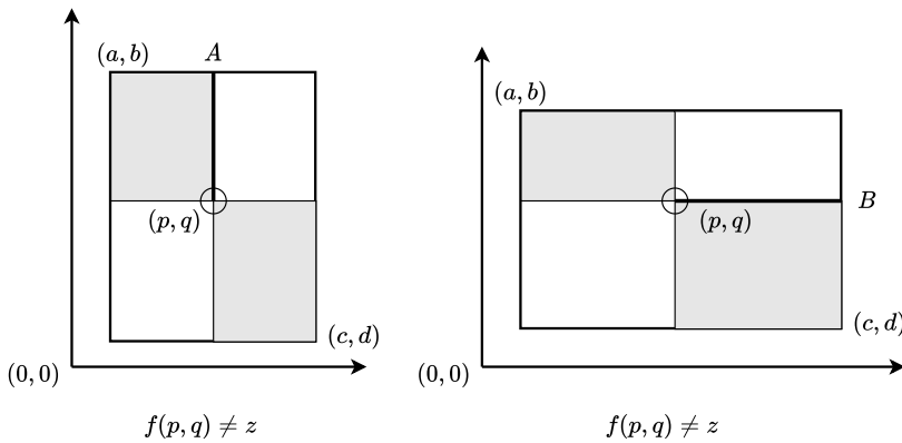
图 14.9: 递归搜索灰色的区域, 如果 f(p, q) \neq z , 还需要搜索加粗的线段。
