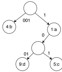
图 6.4: 小端整数树实现的映射 \{1 \rightarrow a, 4 \rightarrow b, 5 \rightarrow c, 9 \rightarrow d\}
