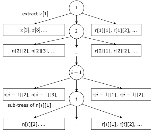
图 12.10: 自底向上遍历,直到提取出一个叶子节点
