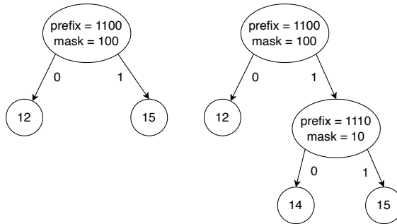
(a) 插入 14 = (1110)_2 , 它和最长公共前缀 p = (1100)_2 匹配, 递归插入右子树。
