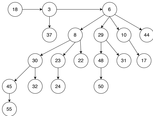
图 10.3: 含有 19 个元素的二项式堆
