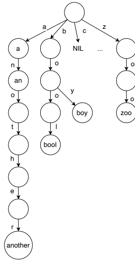
图 6.8: 含有多达 26 个分枝的 trie, 包含键: a、an、another、bool、boy、zoo
