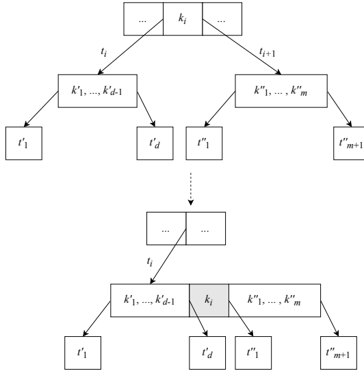
图 7.17: 合并 t_i, k, t_{i+1}
