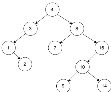
图 2.2: 二叉搜索树的例子
