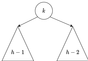
图 5.2: 高度为 h 的 AVL 树, 其中一棵子树高 h - 1 , 另外一棵的高度不小于 h - 2
