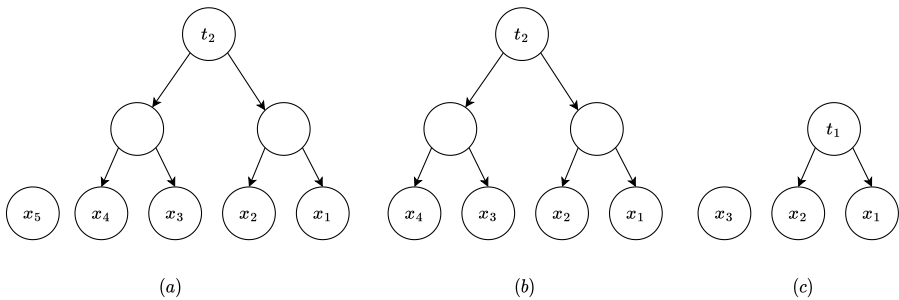
图 12.3: 从头部删除元素: (a) x_1, x_2, \dots, x_5 对应 [t_0, t_2] 。 (b) 删除 x_5(t_0) 。 (c) 删除 x_4 。 经过两次拆分后得到 [t_0, t_0, t_1] , 删除后得 [t_0, t_1] 。
