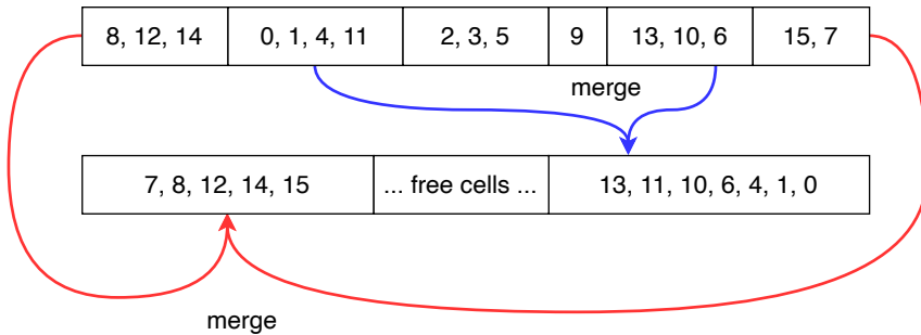
图 13.15: 自然归并排序
