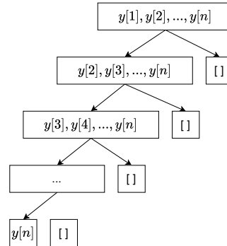
(b) [y_1 > y_2 > \dots > y_n] 的划分树, ≥ p 的部分总为空。
