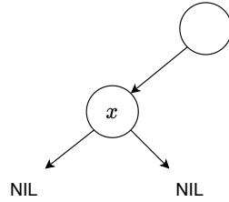
图 2.4: 直接“切掉”叶子节点 x 。
