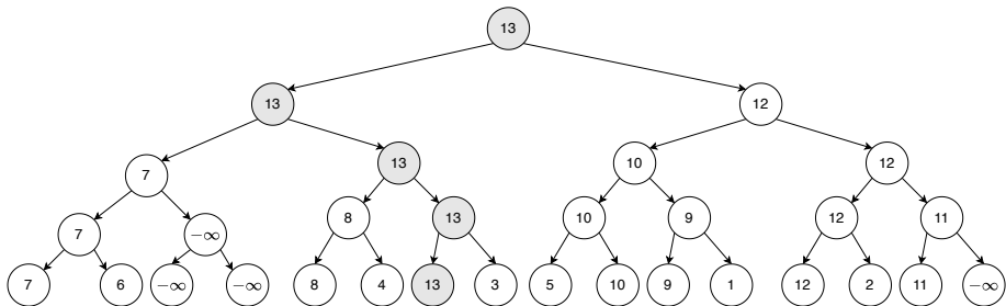
图 9.6: 锦标赛树排序的前几步
