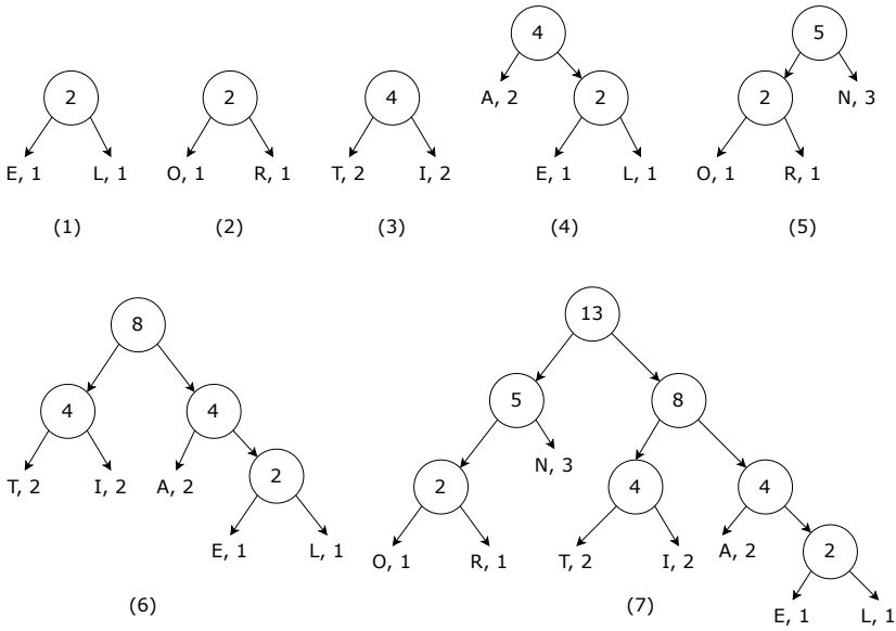
图 15.21: 构造哈夫曼树
