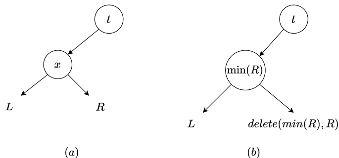
图 2.6: 删除有两个非空分支的节点
