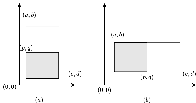
图 14.10: 沿中线二分查找时的特殊情况
