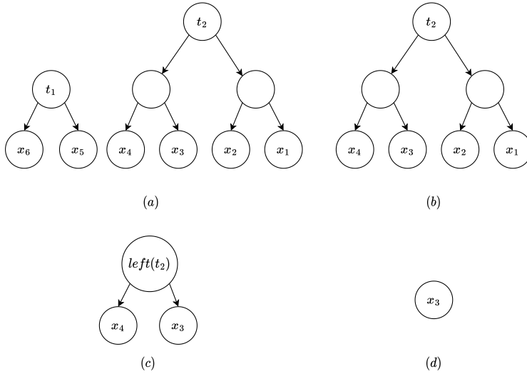
图 12.4: 获取 S[4] : (a) S[4], 4 > size(t_1) = 2 (b) S'[4 - 2] \Rightarrow lookup_T 2 t_2 (c) 2 \leq \lfloor \frac{size(t_2)}{2} \rfloor \Rightarrow lookup_T 2 left(t_2) (d) lookup_T 1 right(left(t_2)) , 返回 x_3 。
