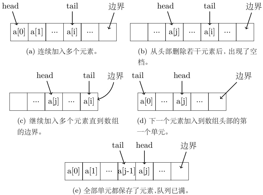
图 11.4: 使用循环缓冲区实现队列
