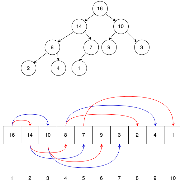
图 8.1: 完全二叉树到数组的映射
