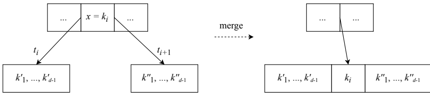
图 7.14: 先合并再删除
