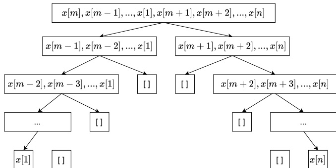
(a) 除了第一次划分,其它都不平衡。
