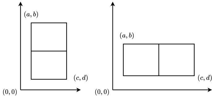
图 14.8: 沿较短的中线二分查找
