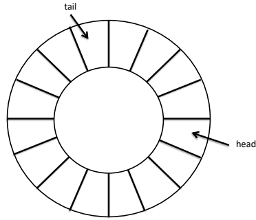
图 11.3: 循环缓冲区
