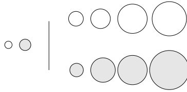
图 13.8: 归并
