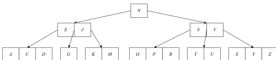
图 7.1: B 树
