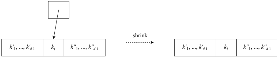
图 7.15: 缩减高度
