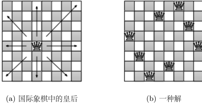
图 15.3: 八皇后问题
