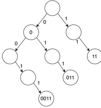
图 6.2: 大端(big-endian)trie
