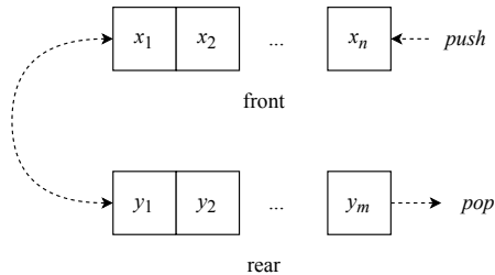
图 11.6: 双数组队列
