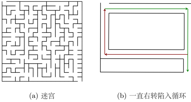
图 15.1: 迷宫
