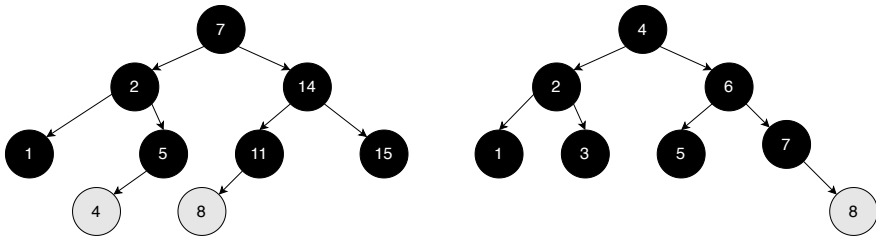
图 4.7: 插入产生的红黑树
