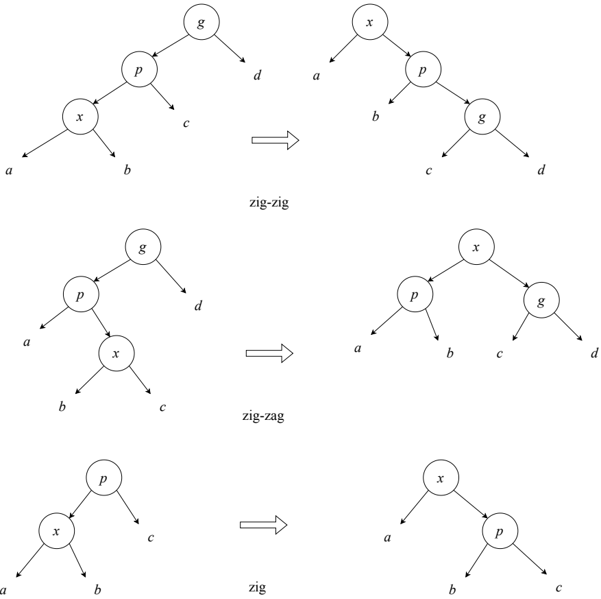
图 8.10: zig-zig : x 和 p 都是左子树或都是右子树, x 成为根节点。 zig-zag : x 和 p 一左一右, x 成为根节点, p 和 g 变成兄弟节点。 zig : p 是根节点, 旋转后 x 变为根节点。
