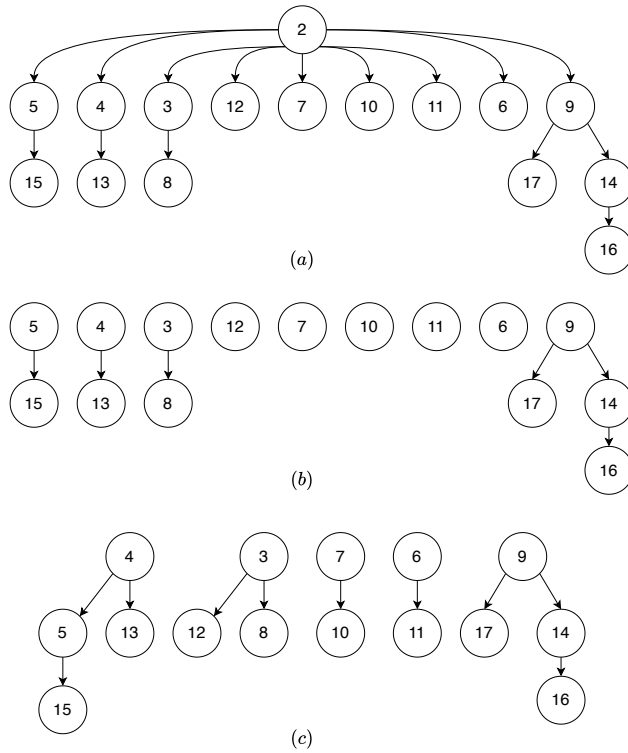
图 10.10: 删除根节点, 将子树成对合并。剩下 9 棵子树中的最后一棵。
