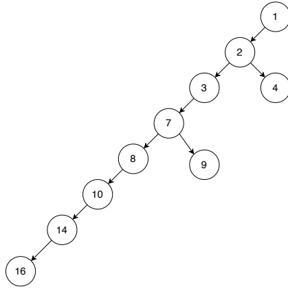
图 8.8: 从序列 [16, 14, 10, 8, 7, 9, 3, 2, 4, 1] 构造的左偏堆
