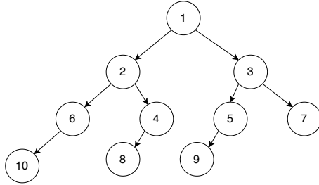
图 8.9: 用已序序列 [1, 2, \dots, 10] 构造的斜树
