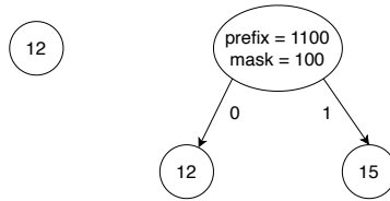
图 6.5: 左: T 是叶子节点 12; 右: 插入 15 后
