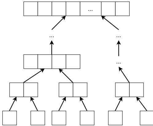
图 13.17: 自底向上归并排序
