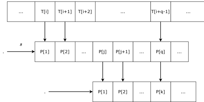
图 14.13: P_k 同时是 P_q 的前缀和后缀
