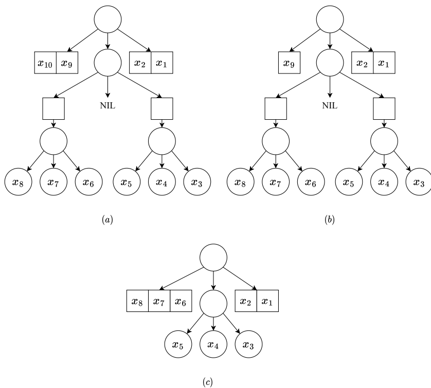
图 12.8: 删除:(a) 含有 10 个元素的树。(b) 删除一个元素后, f 还剩一个元素。(c) 再次删除一个元素, 从中间子树“借”一个节点, 将它从 2-3 树转换成列表, 作为新的 f 。
