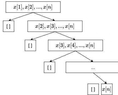
(a) [x_1 < x_2 < \dots < x_n] 的划分树。≤ p 的部分总为空。
