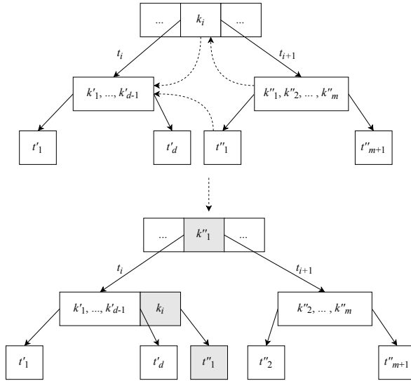
图 7.16: 从右侧移入一个元素
