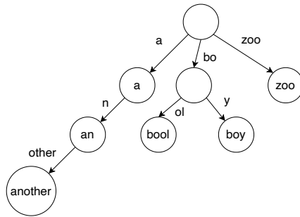
图 6.9: 一棵前缀树, 包含键: a、an、another、bool、boy、zoo
