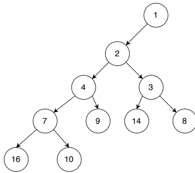
图 8.7: 从列表 [9, 4, 16, 7, 10, 2, 14, 3, 8, 1] 构造左偏堆
