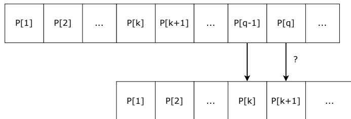
图 14.14: P_k 是 P_{q-1} 的后缀, 比较 P[q] 和 P[k+1]
