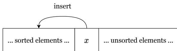
图 3.2: 不断将元素插入已序部分
