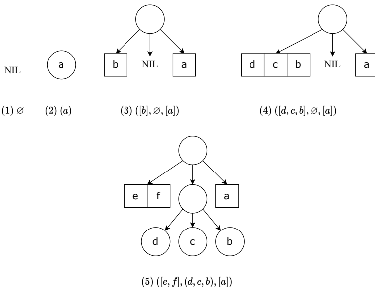
图 12.7: 手指树
