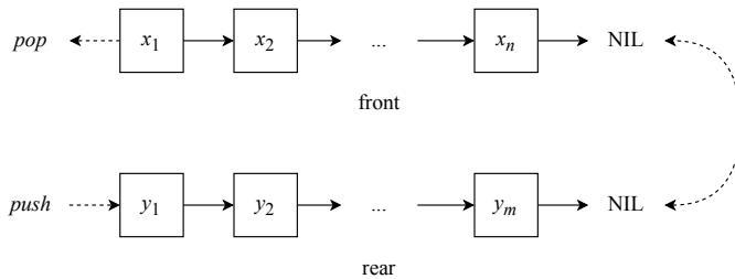
图 11.5: 双列表队列
