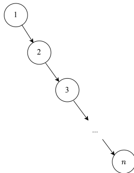
图 4.1: 不平衡的树
