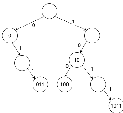
图 6.1: 基数树
