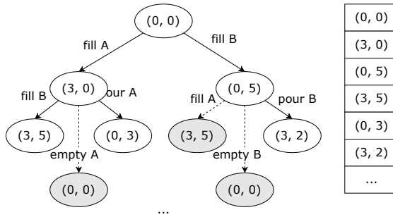
图 15.13: 全局记录
