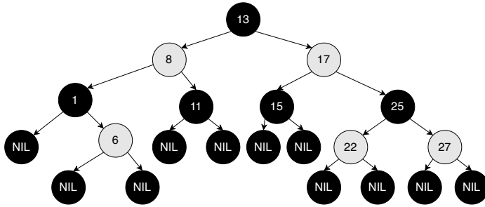
图 4.4: 红黑树
