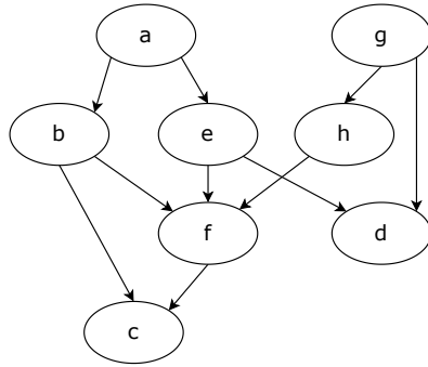
图 15.8: 一个有向图
