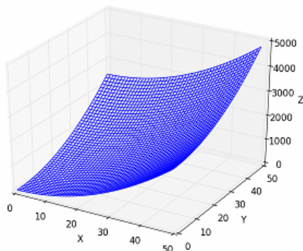
图 14.5: f(x, y) = x^2 + y^2 的图像
