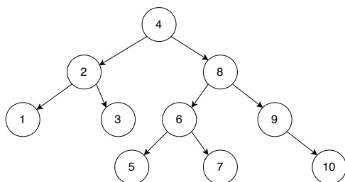
图 5.1: AVL 树
