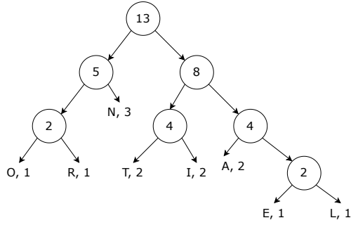
图 15.20: 哈夫曼树
