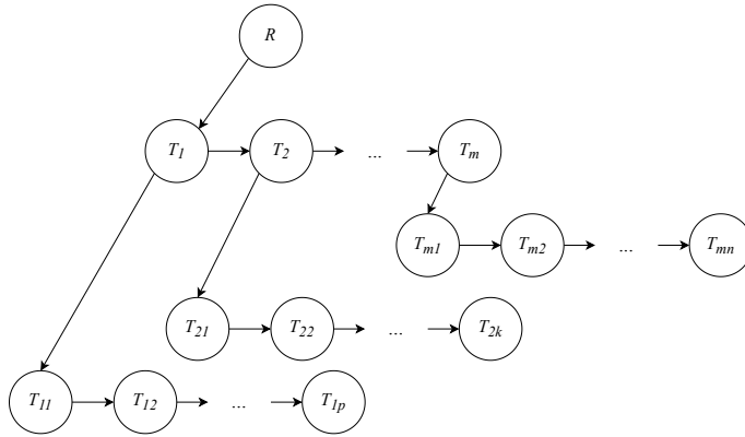
图 10.4: R 为根节点, T_1, T_2, \dots, T_m 为 R 的子树。 R 的左侧为 T_1 , 右侧为空。 T_{11}, \dots, T_{1p} 为 T_1 的子树。 T_1 的左侧是子树 T_{11} , 右侧是兄弟节点 T_2 。 T_2 的左侧是子树 T_{21} , 右侧是兄弟节点。
