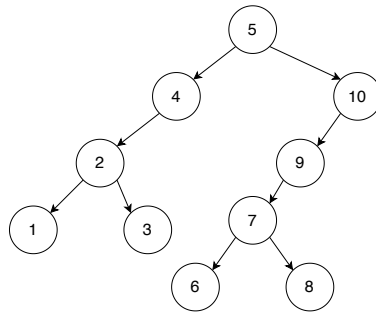
图 8.11: 从 [1, 2, \dots, 10] 产生的伸展树。
