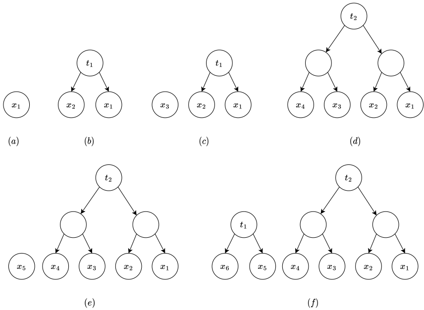
图 12.2: 插入 x_1, x_2, \dots, x_6 : (a) 插入 x_1 。 (b) 插入 x_2 , 链接产生 [t_1] 。 (c) 插入 x_3 , 结果为 [t_0, t_1] 。 (d) 插入 x_4 。 经两次链接后结果为 [t_2] 。 (e) 插入 x_5 , 结果为: [t_0, t_2] 。 (f) 插入 x_6 , 结果为: [t_1, t_2] 。
