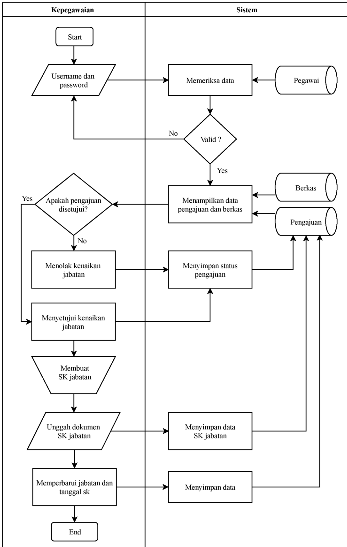
Gambar 5. Flowchart Persetujuan Kenaikan Jabatan dan Pembuatan SK Kenaikan Jabatan
