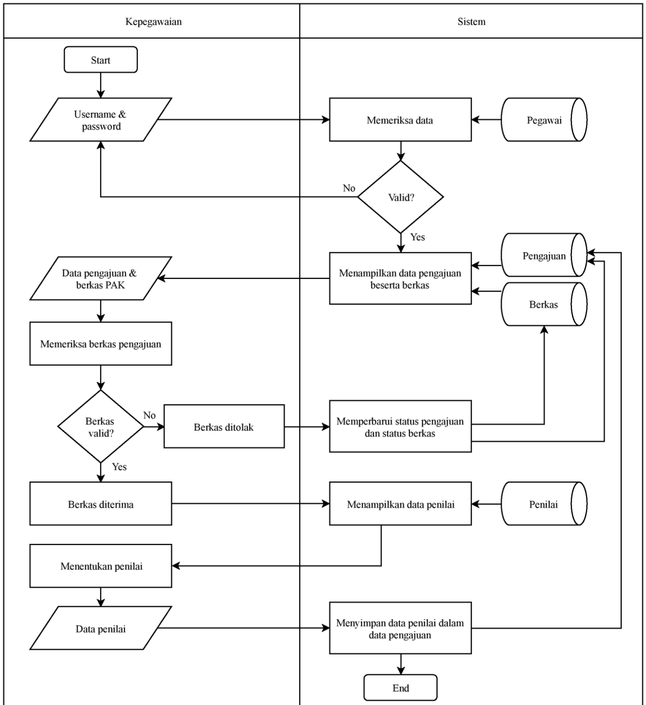
Gambar 3. Flowchart Pemeriksaan Berkas
