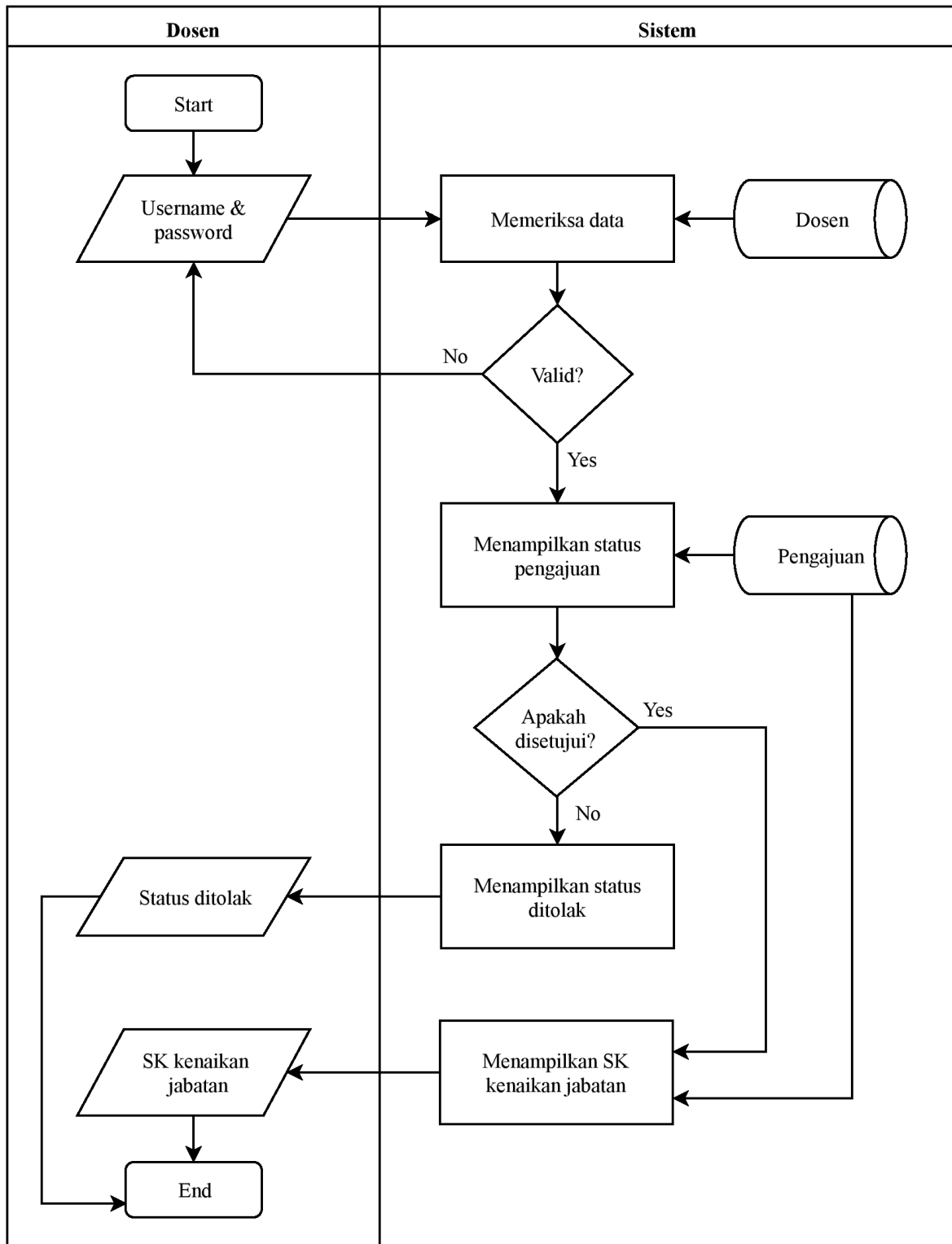
Gambar 6. Flowchart Pemberian Hasil Pengajuan
