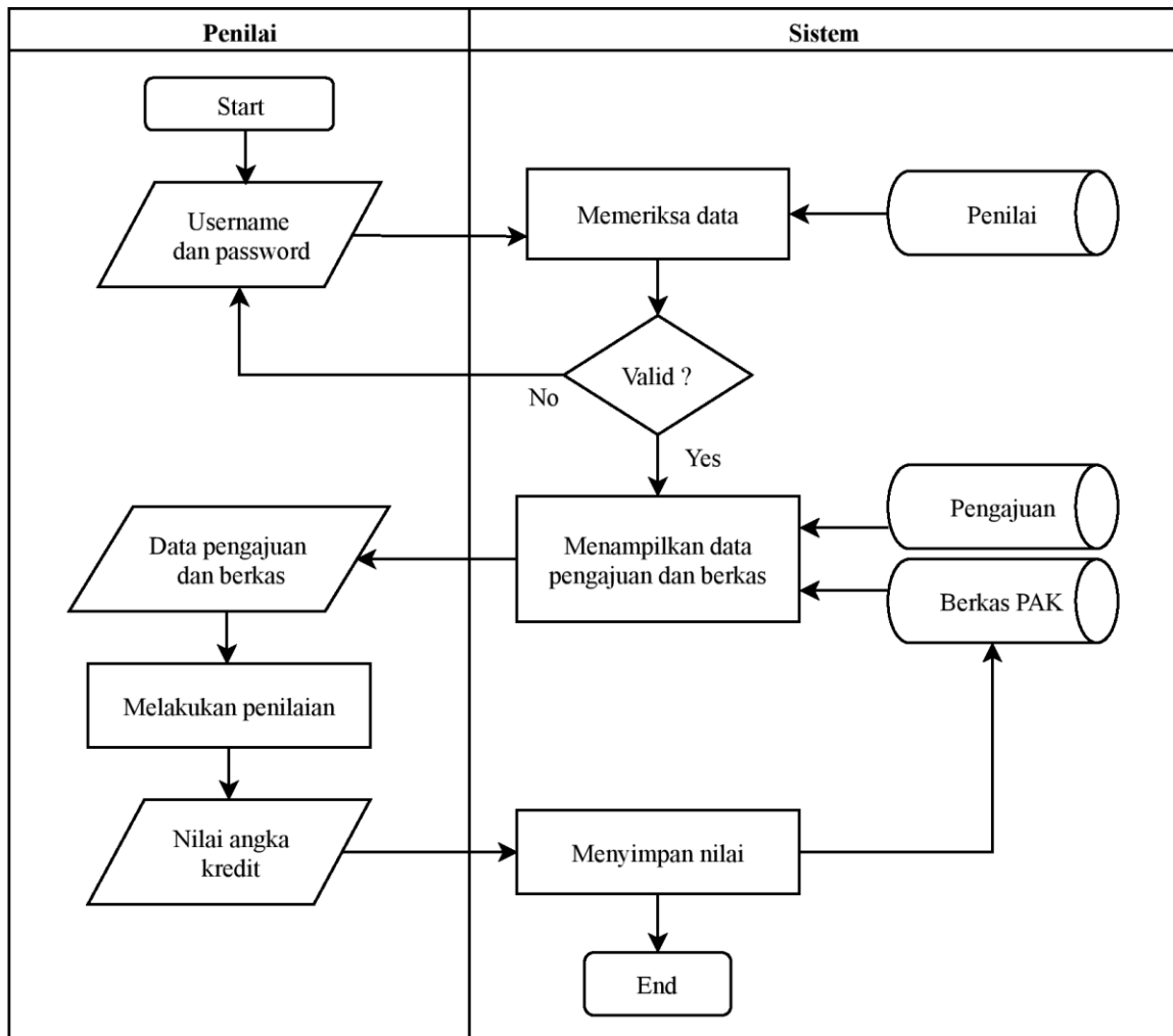
Gambar 4. Flowchart Penilaian Angka Kredit
