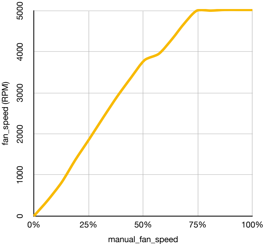
Noctua NF-A4x20 PWM
