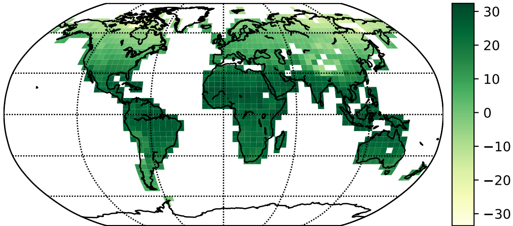
FATES_TVEG [C]
